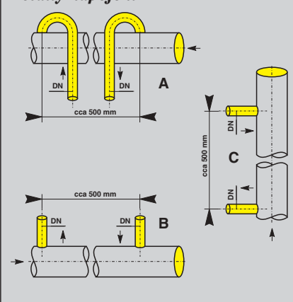
Detaily napojení
